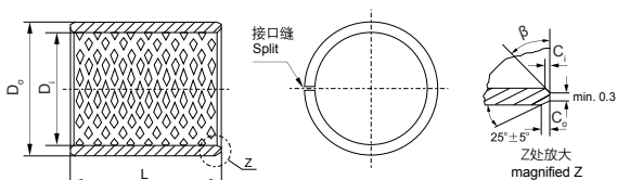
ID and OD chamfers
